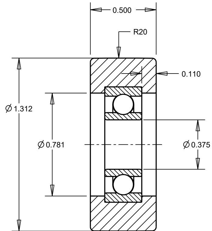
SECTION A-A
