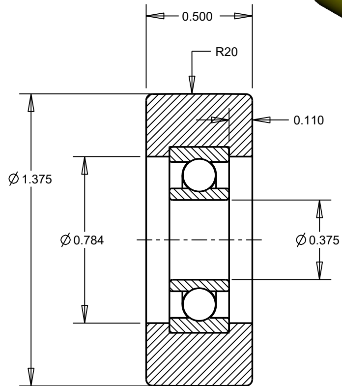
SECTION A-A
